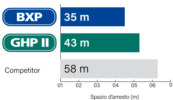
Spazio d'arresto da 60 km/h a 0 - condizione asciutto
