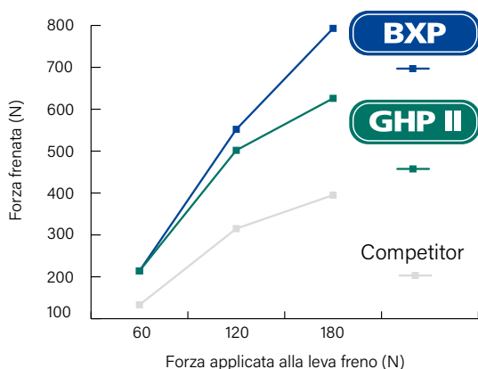
Forza leva vs Forza freno
