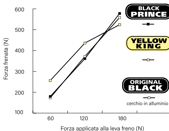
Forza leva vs Forza freno
